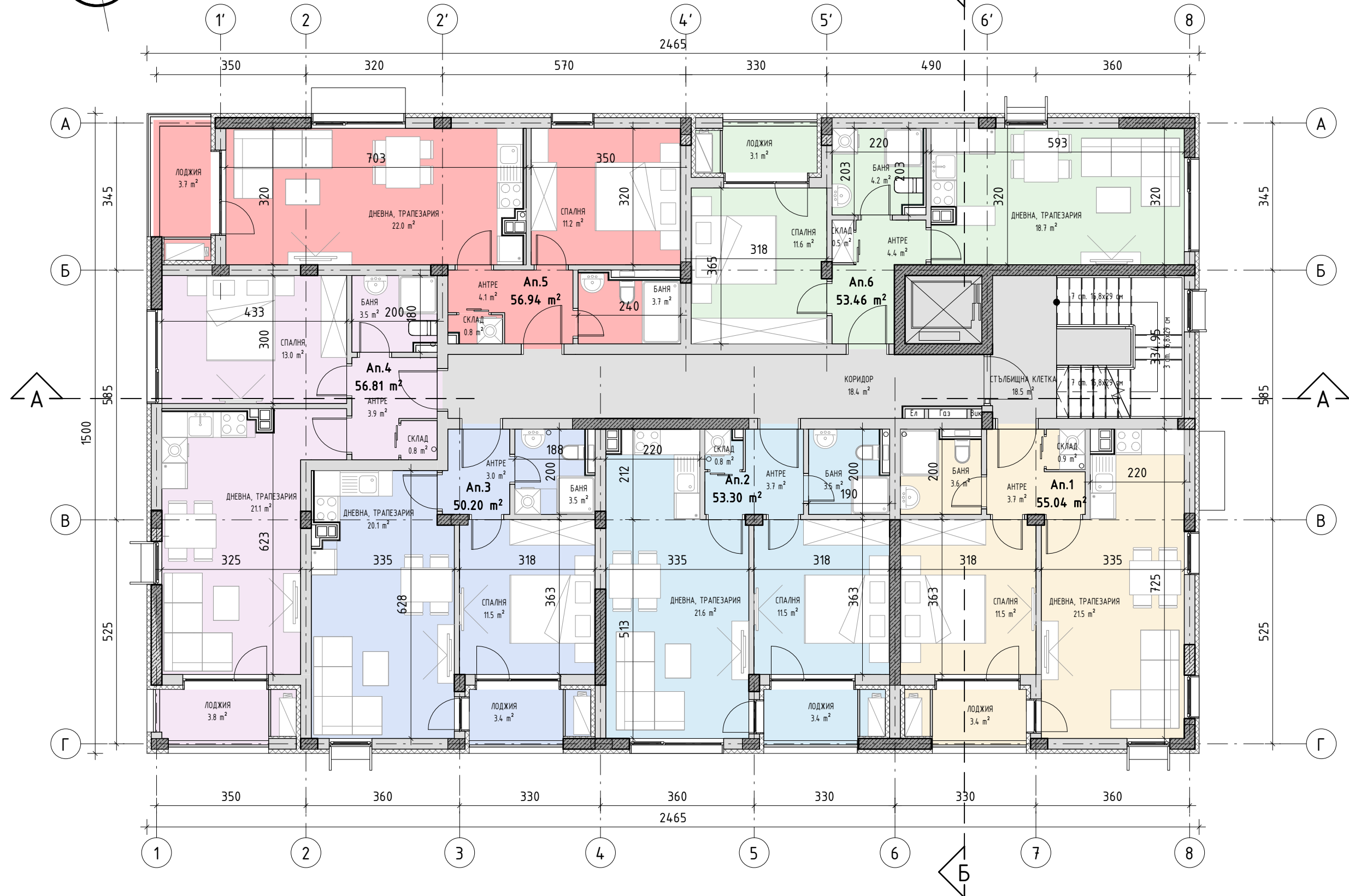
РАЗПРЕДЕЛЕНИЕ КОТА +3.45 М 1:100
